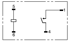
(线圈无极性)
