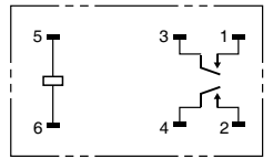
(线圈无极性)
