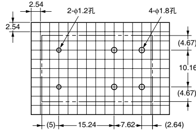
(线圈无极性)
